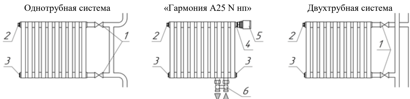
Рис. 2. 1. Вентиль. 2. Кран Маевского-воздухоотводчик. 3. Пробка глухая. 4. Встроенный термодиффузионный клапан. 5. Термостатический элемент. 6. Запорно-присоединительный клапан нижнего подключения.
