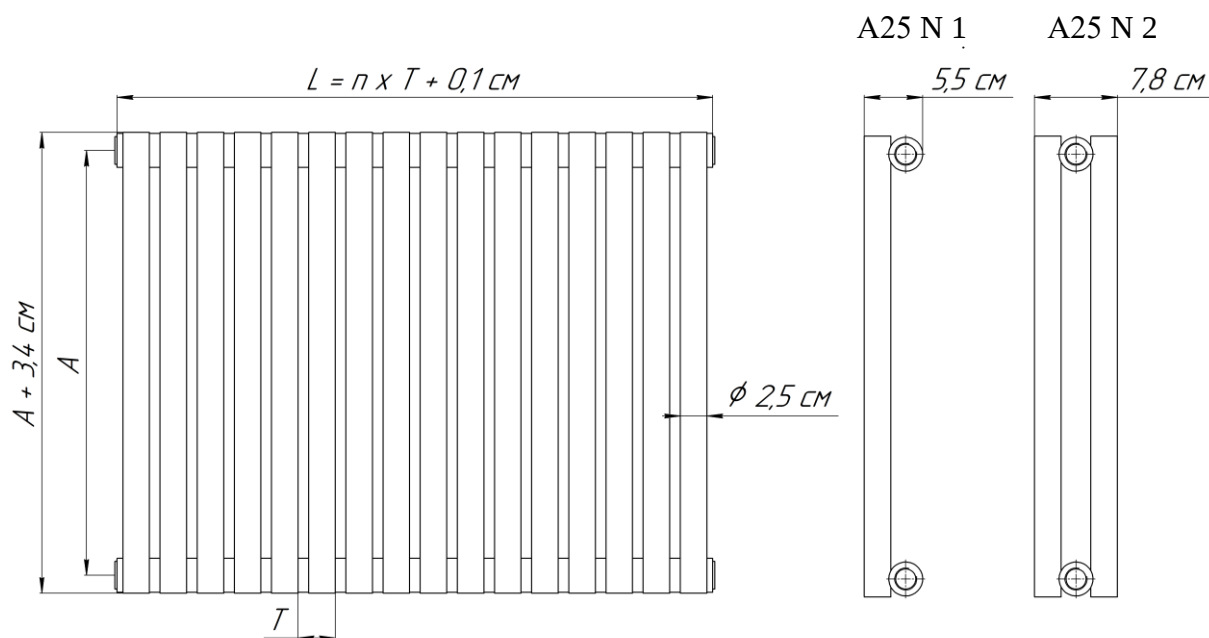
Рис 1. Радиатор «Гармония A25N», где: А – межцентровый размер, см; Т – шаг (Т = 3,5 см); n – количество секций; L – габаритная длина, см.
